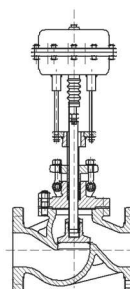
Pneumatický pohon Pneumatic actuator
